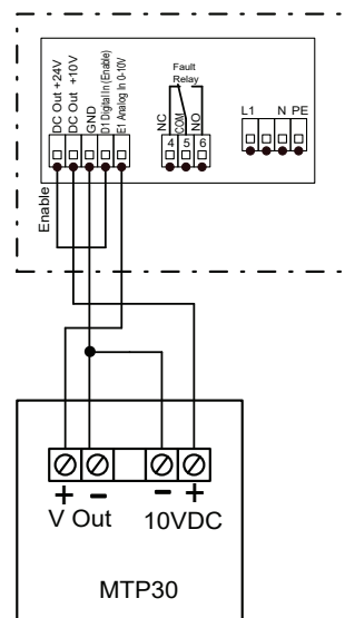
Anschluss Potentiometer MTP30
